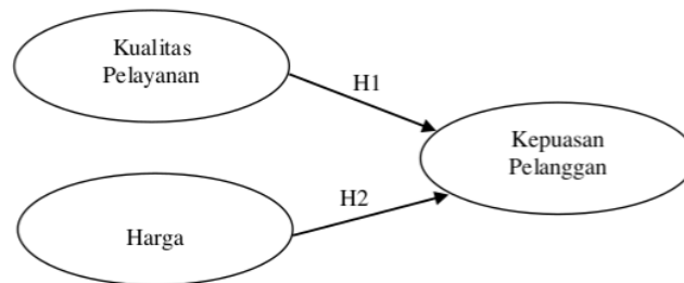
Gambar 1 Kerangka Konseptual
