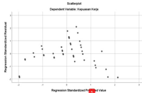
Gambar 2. Uji Heteroskedastisitas
